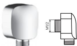
Угловой настенный коннектор для вывода душевого шланга STORM WE-01
