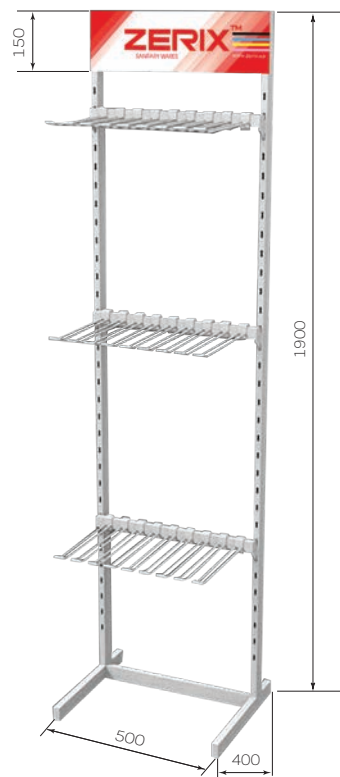
СТЕНД ВИСТАВКОВИЙ під гнучке підведення на 27 гачків 1900×500 мм
