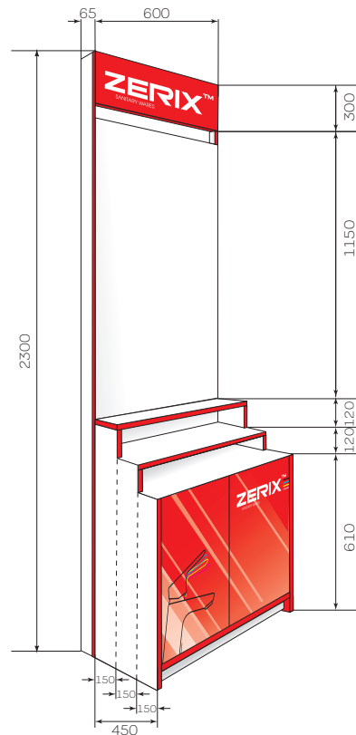
СТЕНД ZERIX 2300×600 мм
